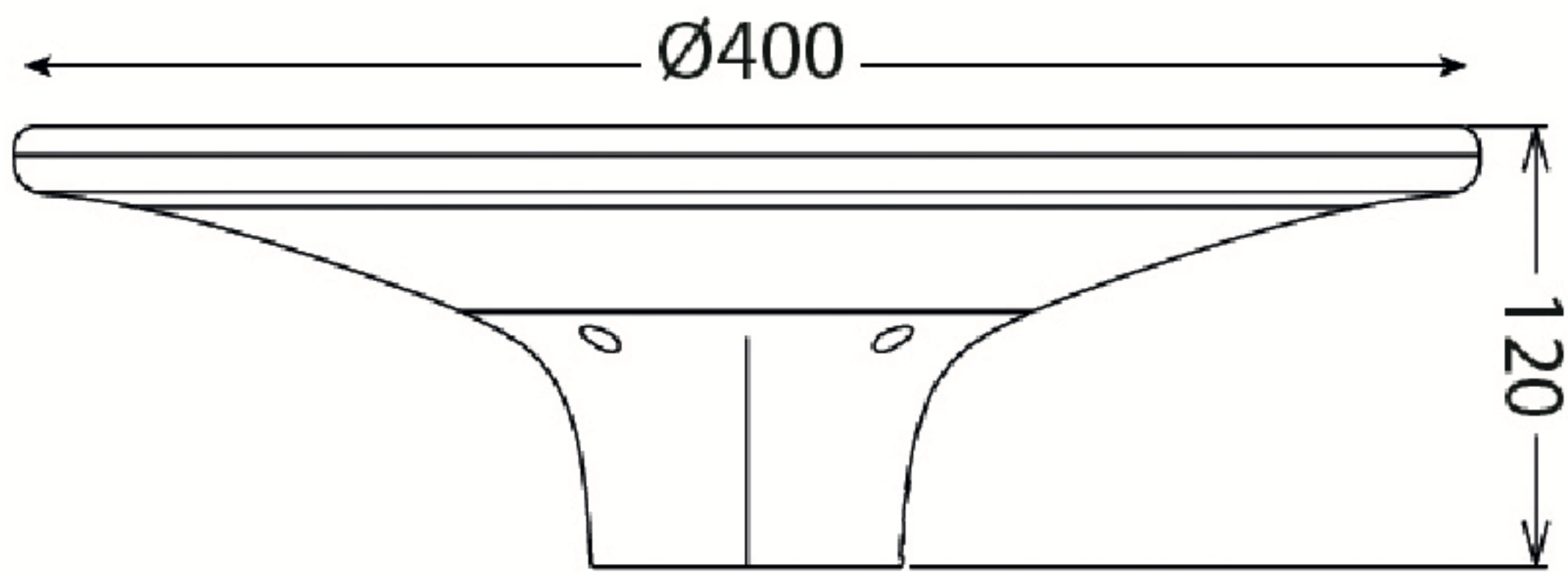
Attacco per palo da Ø60 (palo non incluso)
